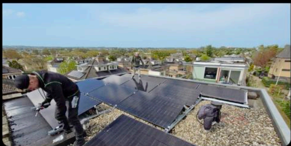
Hybrid-Wechselrichter, Hochvolt-Batterie Rotterdam, Niederlande, Anlagenleistung 10 kW
