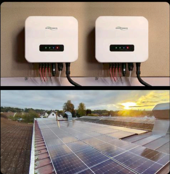
String-Wechselrichter Eure-et-Loir, Frankreich, Anlagenleistung 45 kW
