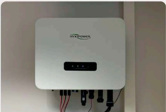
Inversor híbrido Batería de alta tensión Comunidad de Madrid, España Capacidad 5.28kW
