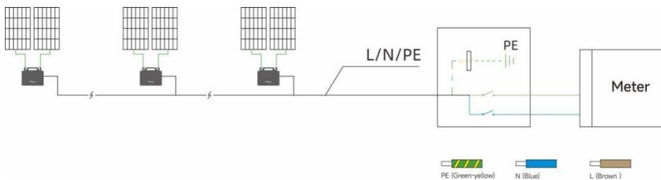
230V Monofase Mappa della messa a terra
