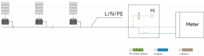
230V Monofase Mappa della messa a terra
