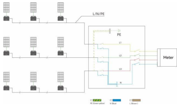
230VAC/400 VAC Mappa di messa a terra trifase
